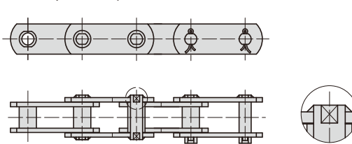
5.销轴铆头后采用焊接加固
